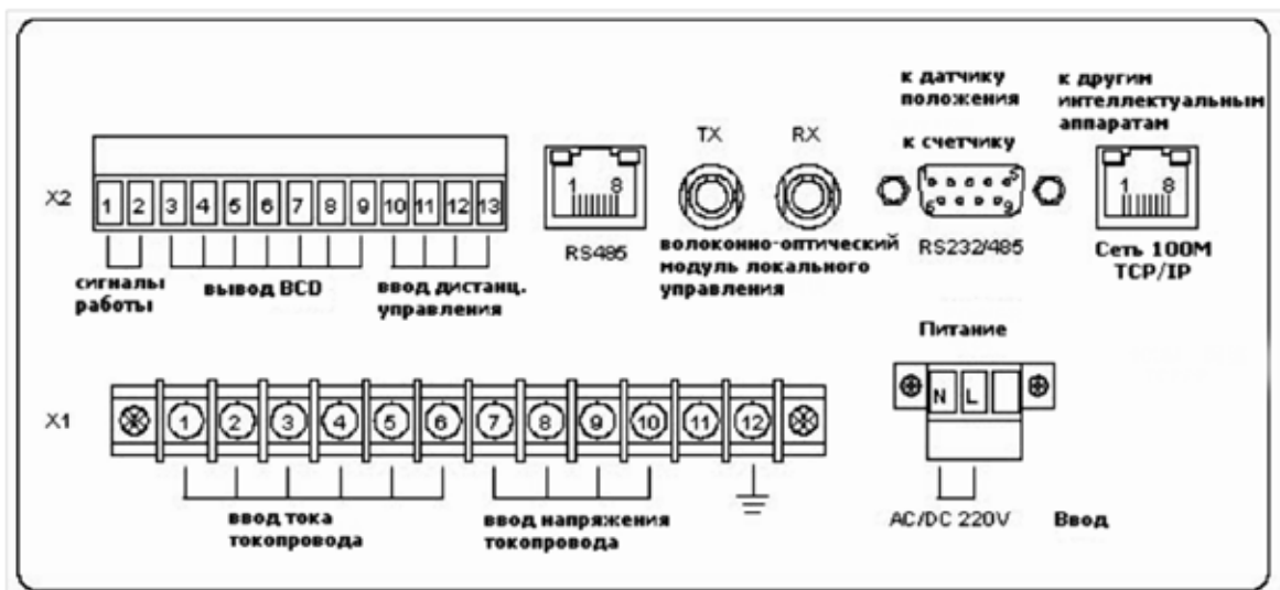
Рис. 6 Задний панель контроллера SHM-K
