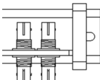
Рис. 5 Разъем CX привода
